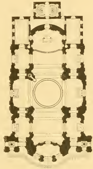
Fig. 63. Kollegienkirche zu Salzburg Grundriß
